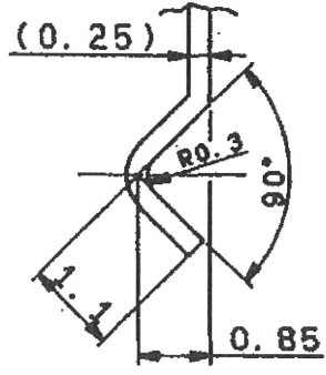
A部詳細 (SCL. 10/1)
